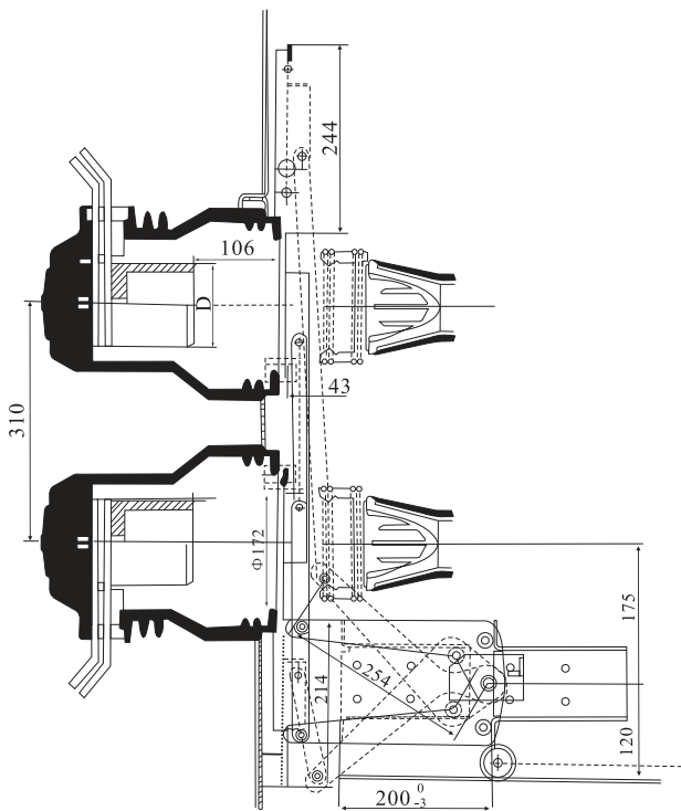
СХЕМА 12. НОМИНАЛЬНЫЙ ТОК 1600–2000 И 2500–5000
