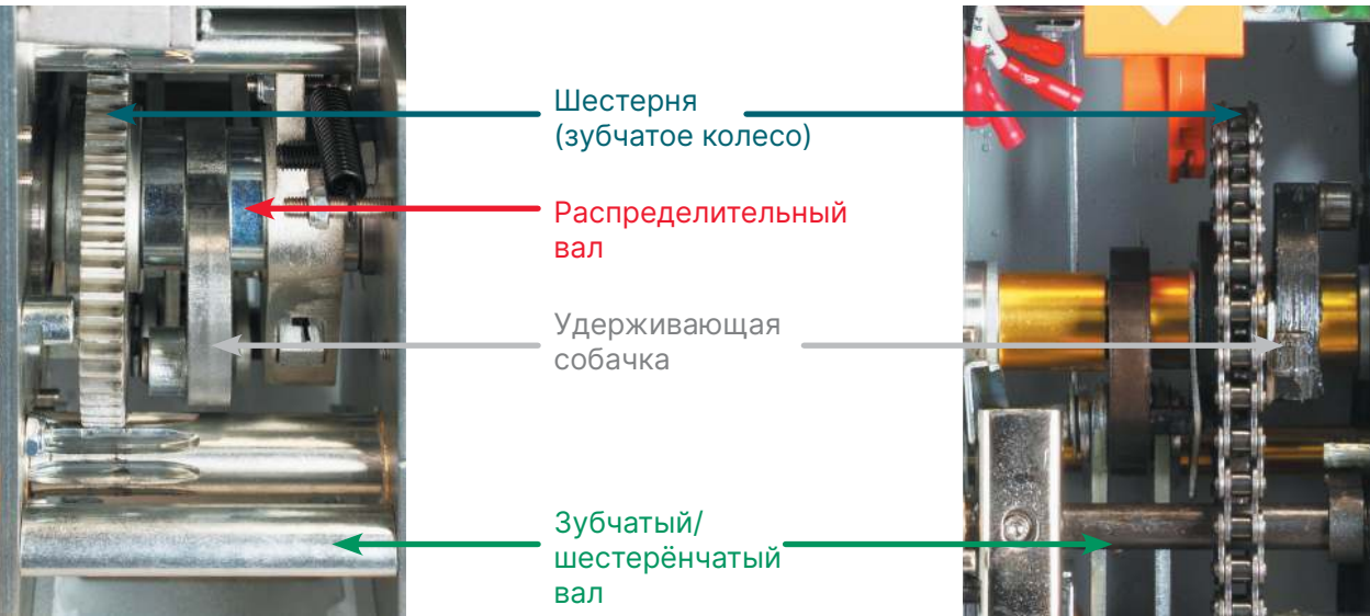
РИСУНОК 7. МЕХАНИЗМ ПЕРЕДАЧИ
