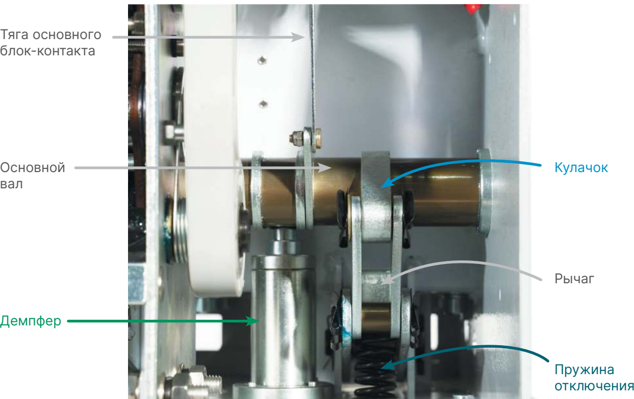
РИСУНОК 8. МЕХАНИЗМ ОТКЛЮЧЕНИЯ
