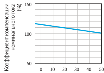
Температура наружного воздуха (при опорной температуре 50°C)
