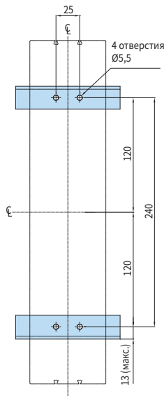
Монтажный чертеж
