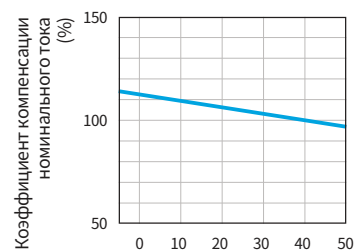
Температура наружного воздуха (при опорной температуре 40°C)
