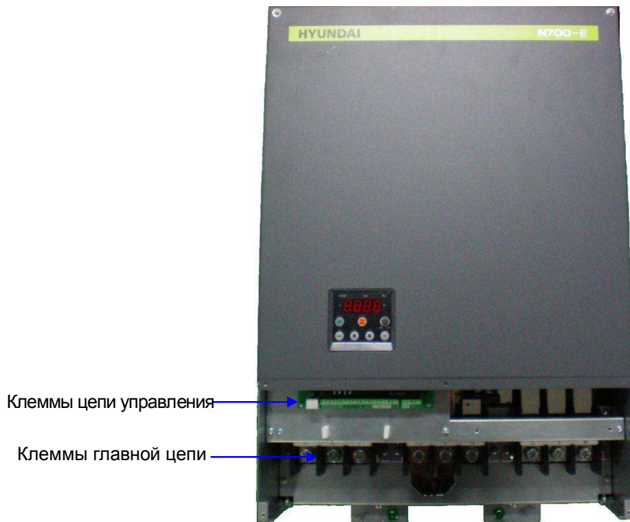
Рис1-6 Передняя крышка снята
