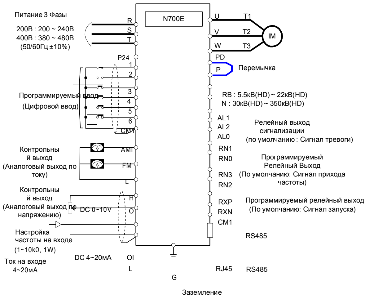
Рис 3-1 Диаграмма настроек от управляющего устройства
